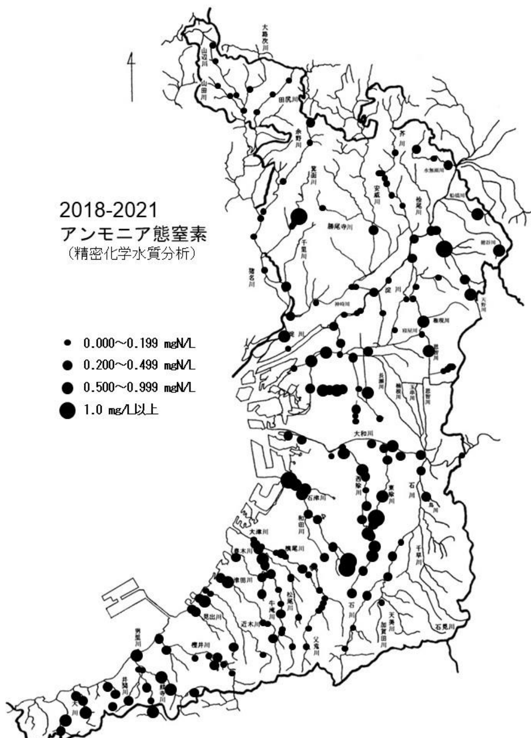
図 3.2.6 精密分析によるアンモニア態窒素
